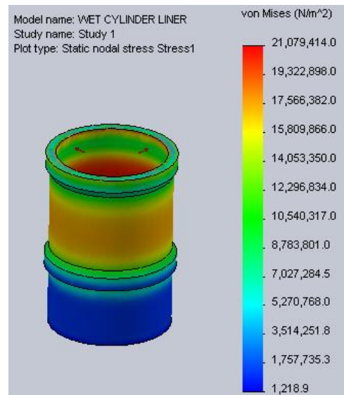
Fig 7: Von Miss Stress
