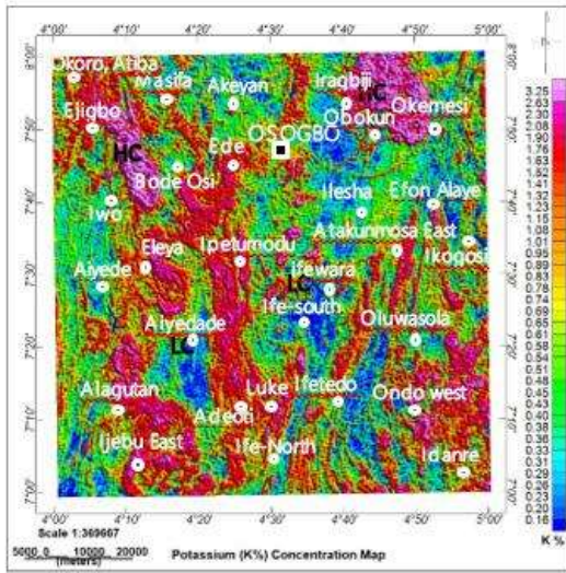
Fig. 7a. Potassium concentration map (K %)
