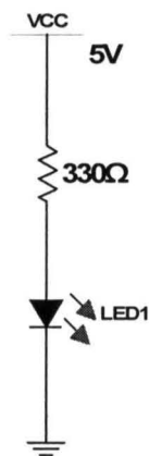
Fig. 3.8 Indicator unit.
