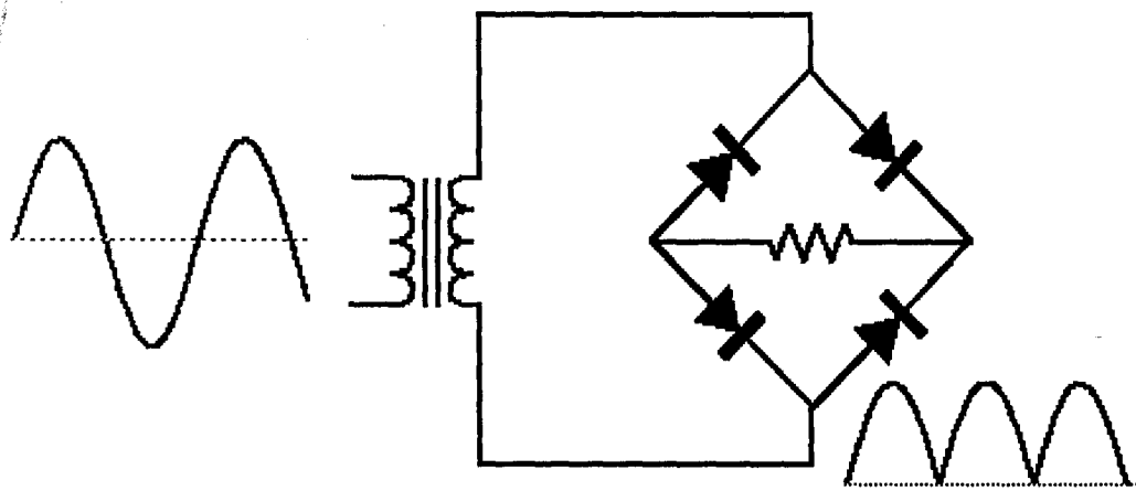
Fig. 3.4 Bridge rectifier
