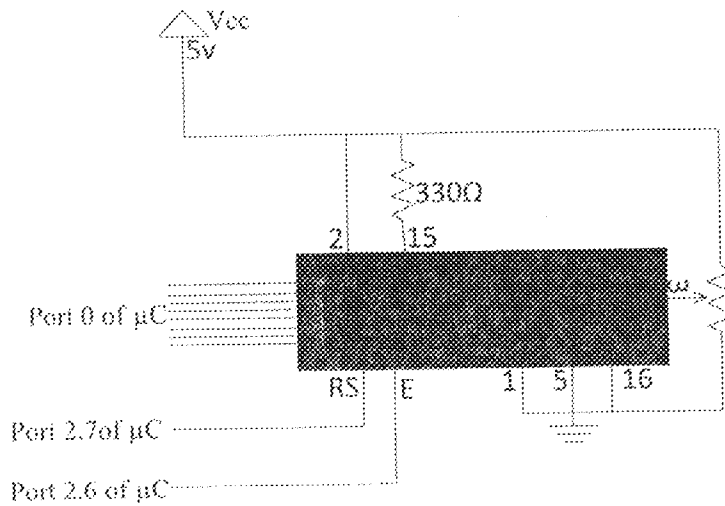
Fig. 3.13 Display Unit
