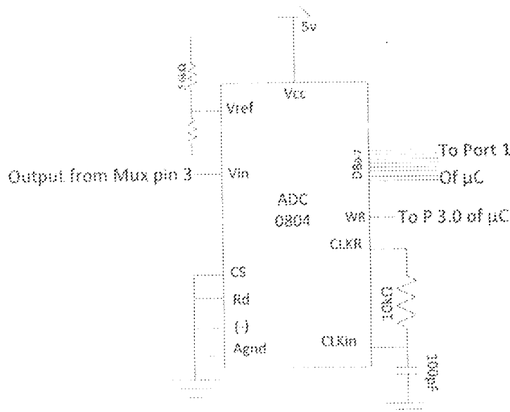
Fig. 3.10 ADC Unit
