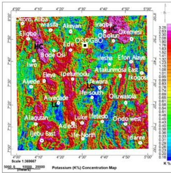
Fig. 7a. Potassium concentration map (K %)
